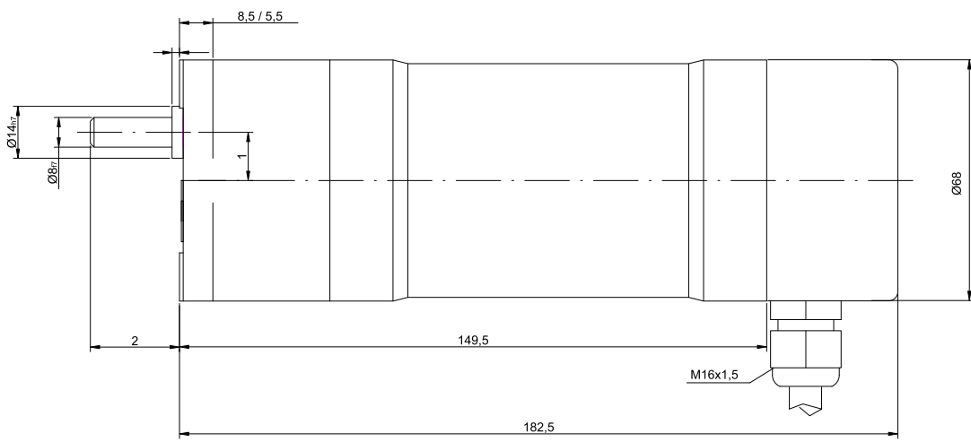
Anschlußleitung: Öfflex-FD Classic 810P 4G 1,0
